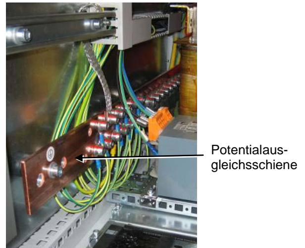
Abbildung 4.13 PE Anschluss
