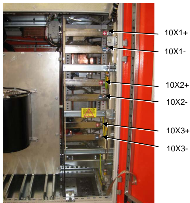
Abbildung 4.11 Leistungsanschlüsse PV-Eingang
