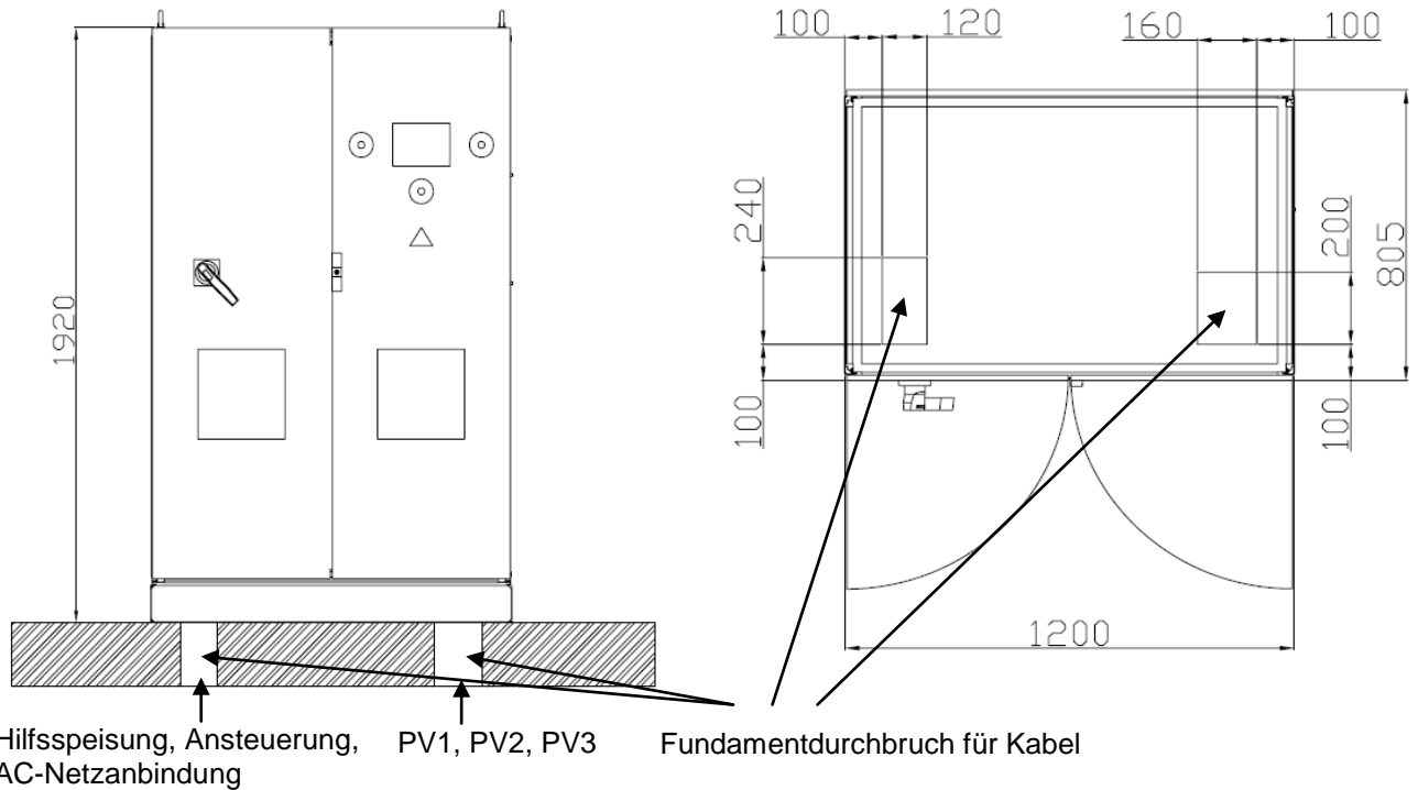
Abbildung 4.3 Fundament
