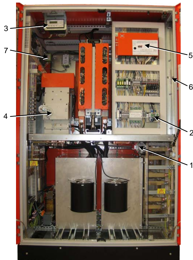
Abbildung 5.3 Wichtige Komponenten
