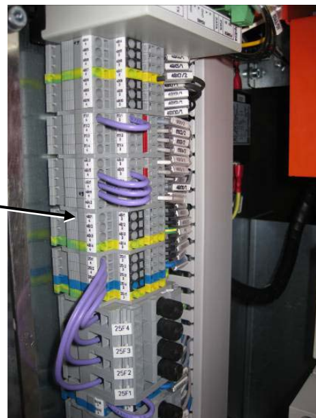
Abbildung 4.15 Vergrößerung der Hilfsklemmen
