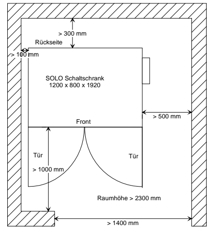
Abbildung 4.2 Mindestabstände
